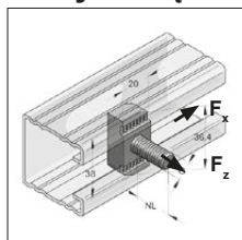
Płytki zębata z bolcem
